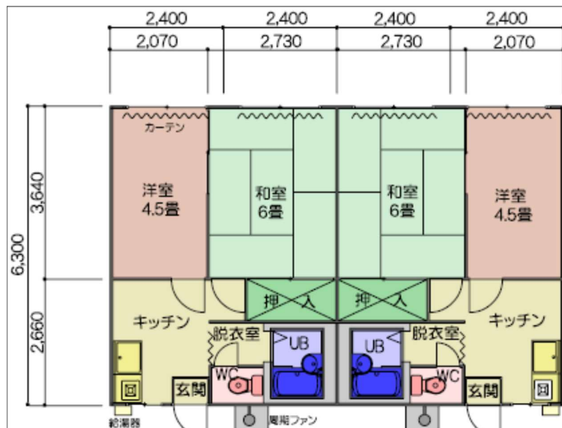
恵南豪雨被害【岐阜県上矢作町】応急仮設住宅標準平面プラン ユニットタイプ（30.2㎡）
