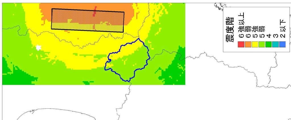
■ 想定地震の震度分布（4 北上低地断層帯、5 新庄盆地断層帯、6 山形盆地断層帯、7 北由利断層帯）
